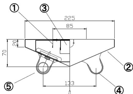
姿図
