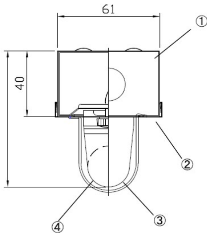
姿図
